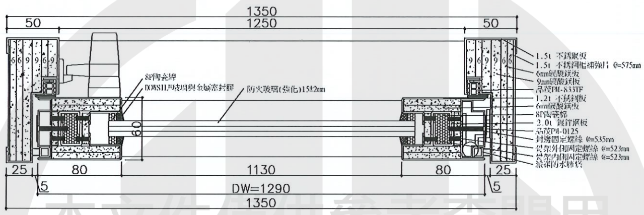
水平剖面圖 單位 mm
