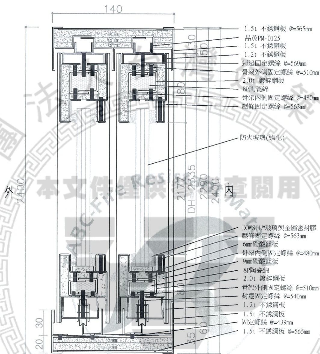
垂直剖面圖-1 單位 mm
