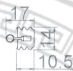
INFS1400組合式防撞型防煙條詳圖
