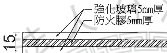
防火玻璃剖面圖
