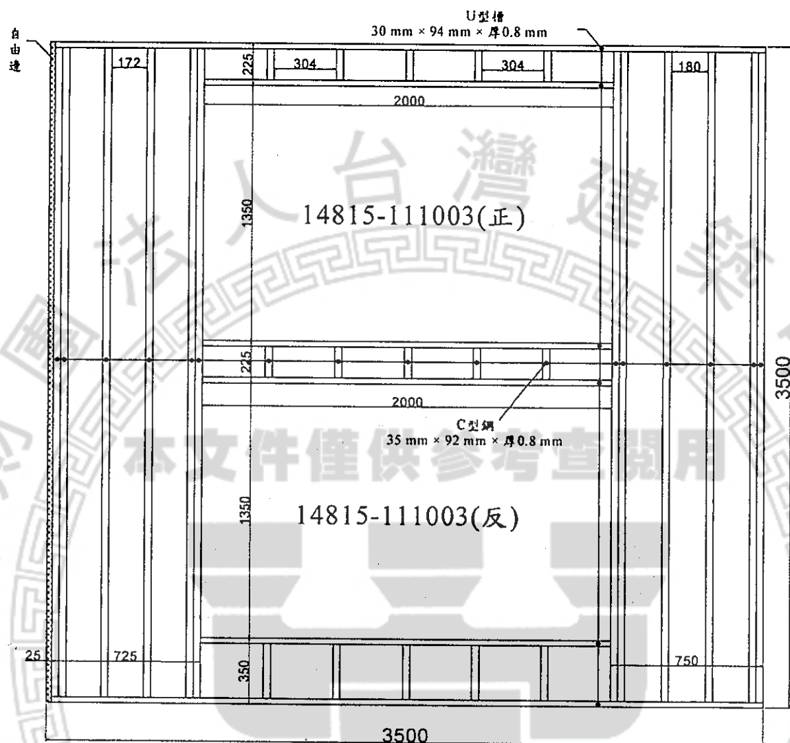
支撐構造圖 單位 mm
