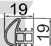
防煙條詳圖
