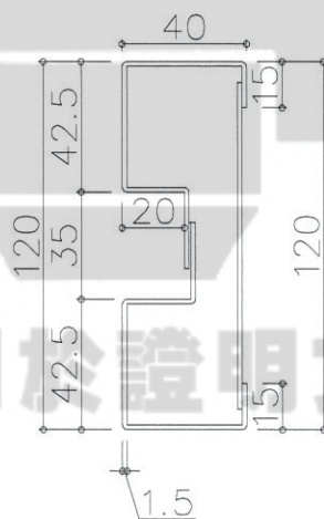
邊框料尺寸詳圖
