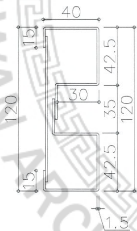
邊框料尺寸詳圖
